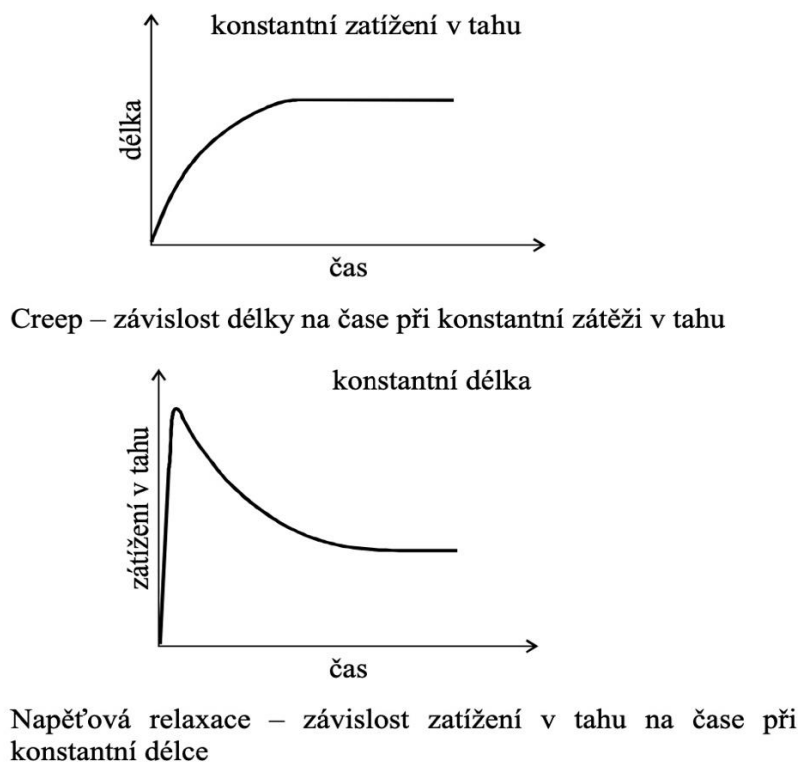
Obrázek 3. Creep a napěťová relaxace (Janura, 2011)
