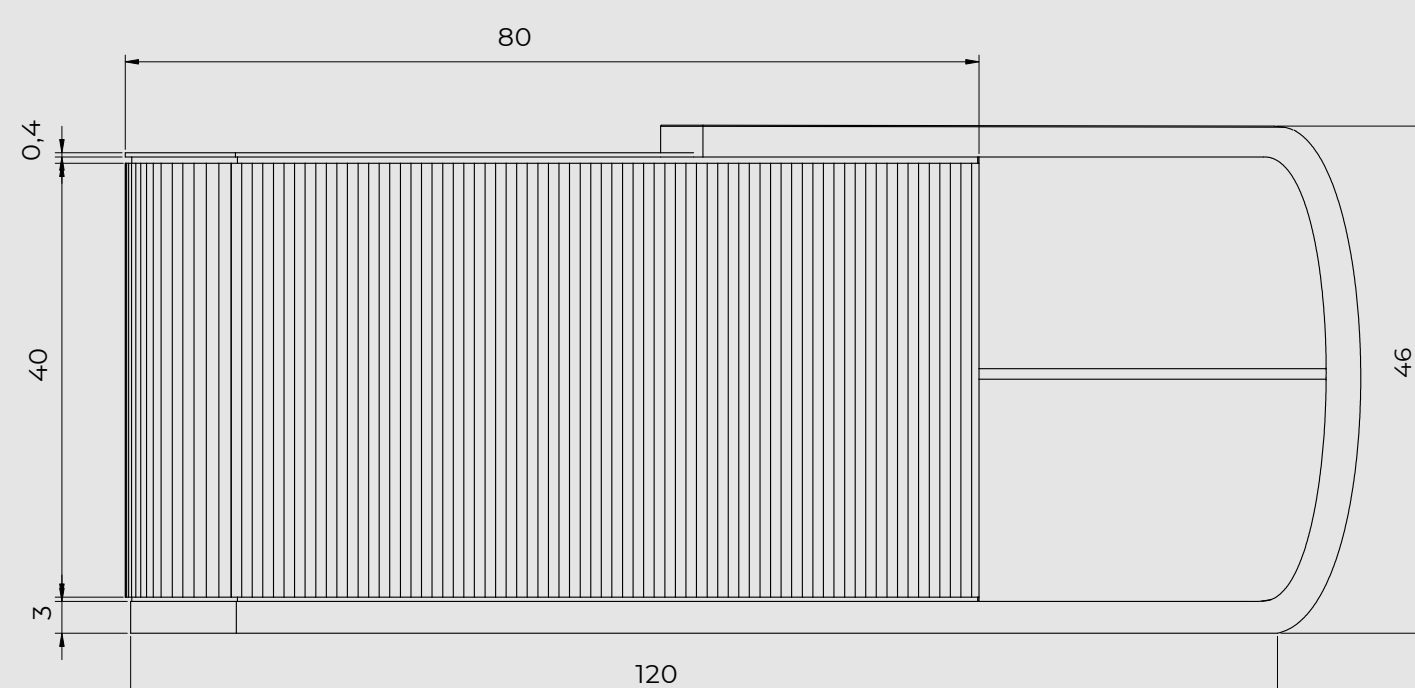
Pohled zepředu
