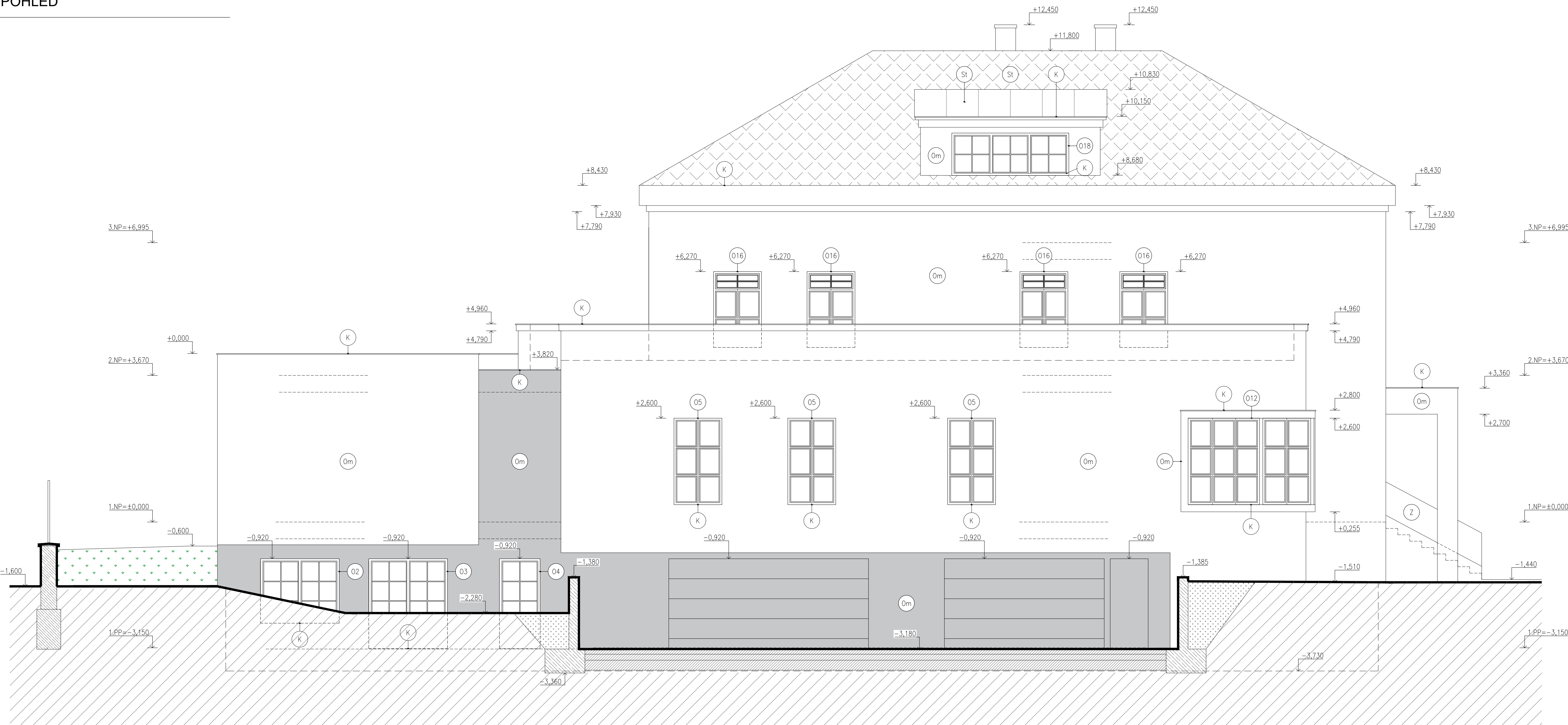
SEVEROZÁPADNÍ POHLED
